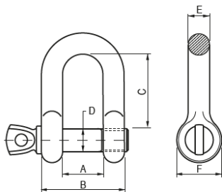
Medidas / Dimensions
